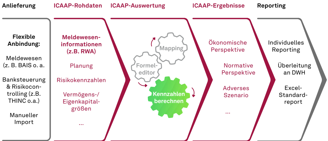
Abbildung 1: Die Funktionsweise von THINC.ICAAP auf einen Blick
